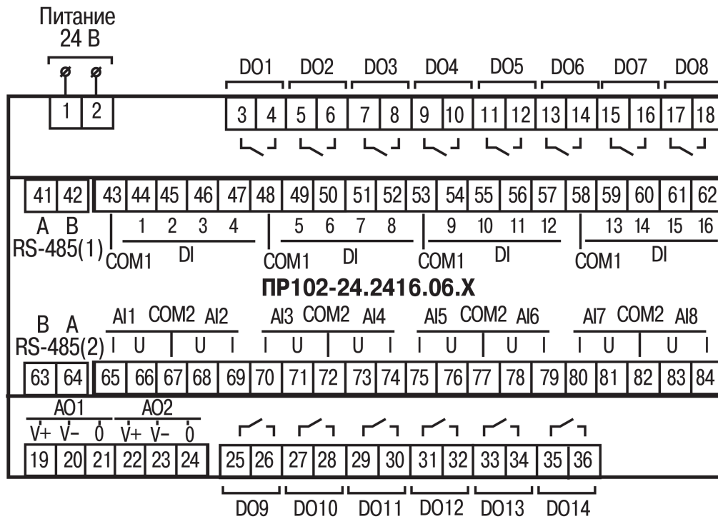
Рисунок А.5 – Расположение контактов для PR102-24.2416.06.X
