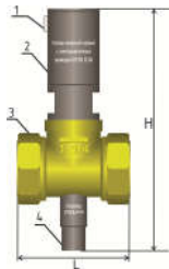
Рисунок 1. Клапан КЗГЭМ-Б.
