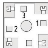
Рисунок Г.8 – Схема подключения клапана КЗЭУГ с разъемом TJ1A-6P6C
