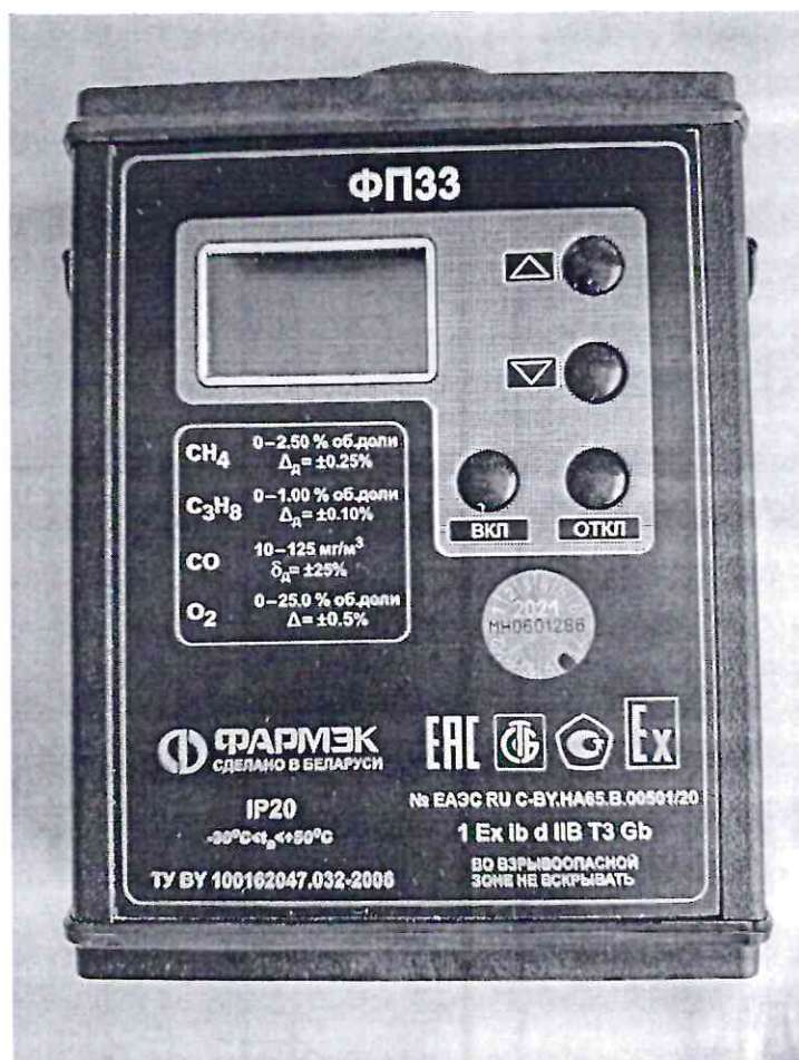
Рисунок 1.1 – Внешний вид газоанализатора
