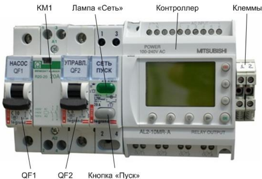
Рис.2 Элементы блока управления.
