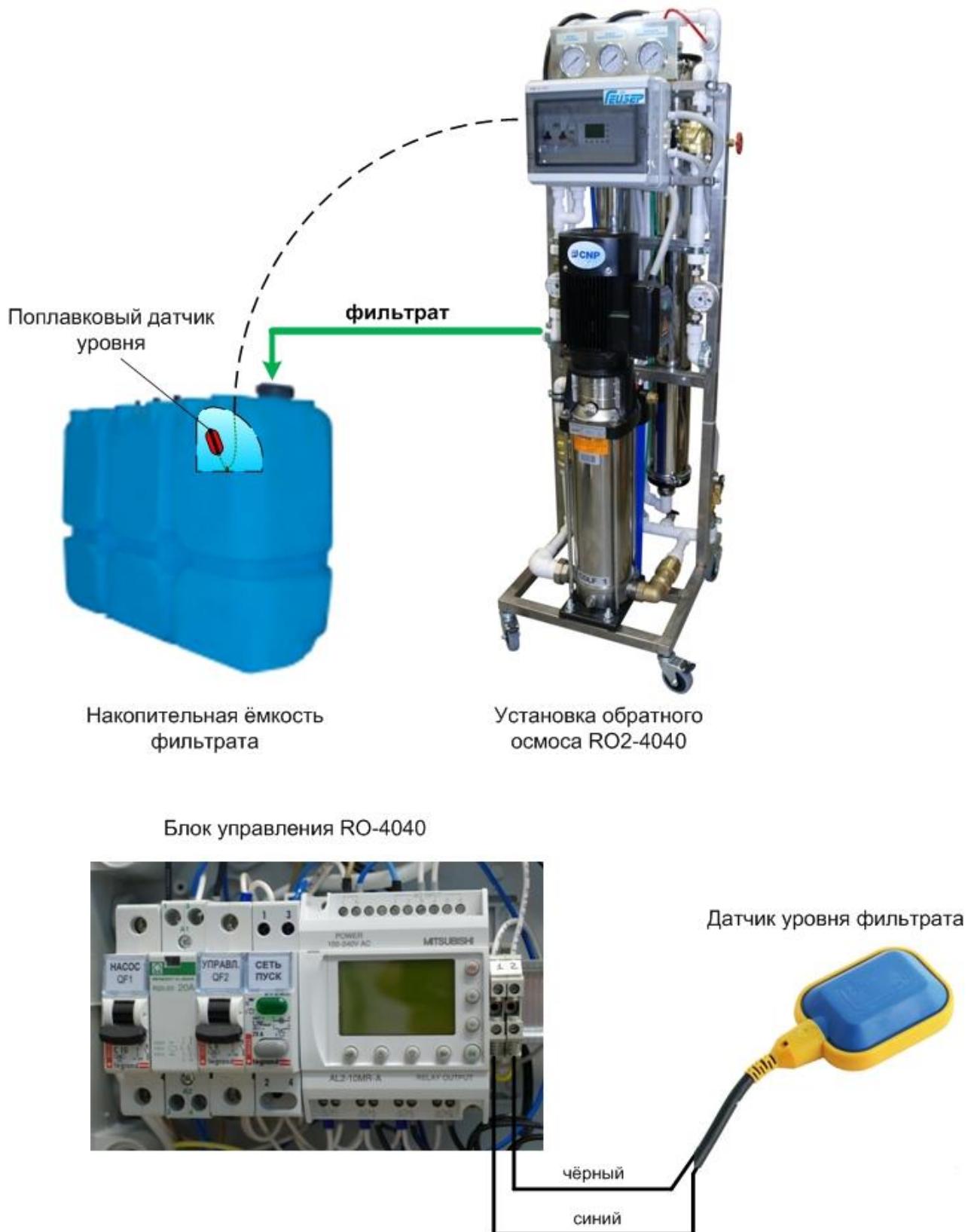
Рис. 5 Подключение одного датчика уровня к установке.
