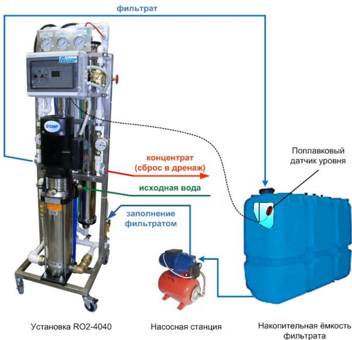
Рис. 4 Подключение трубопроводов к установке.
