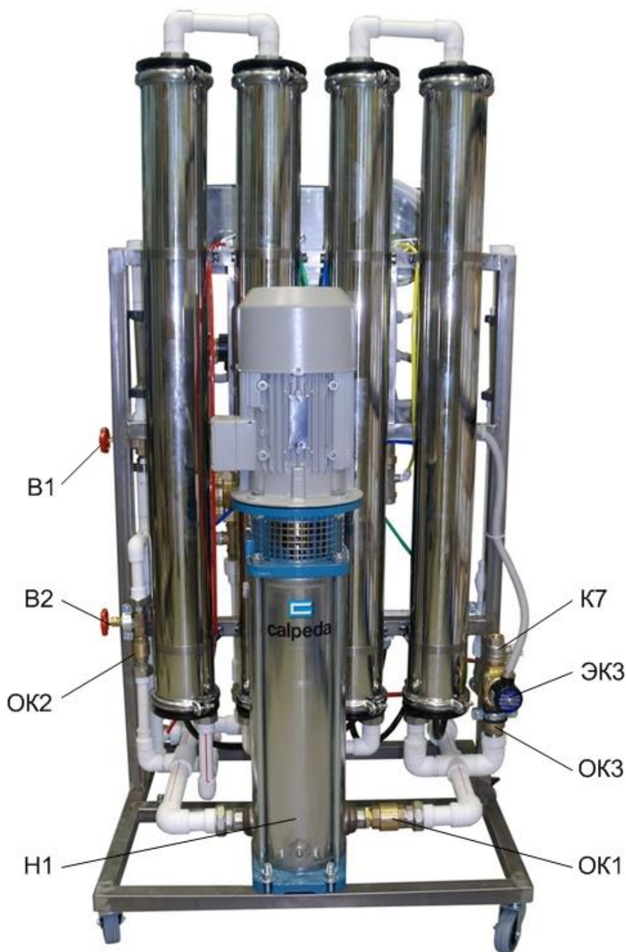
Рис.2 Общий вид установки (со стороны насоса).
