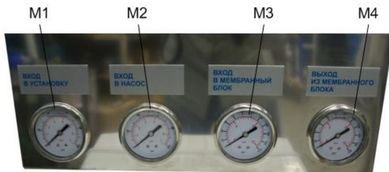
Рис.4 Манометры.
