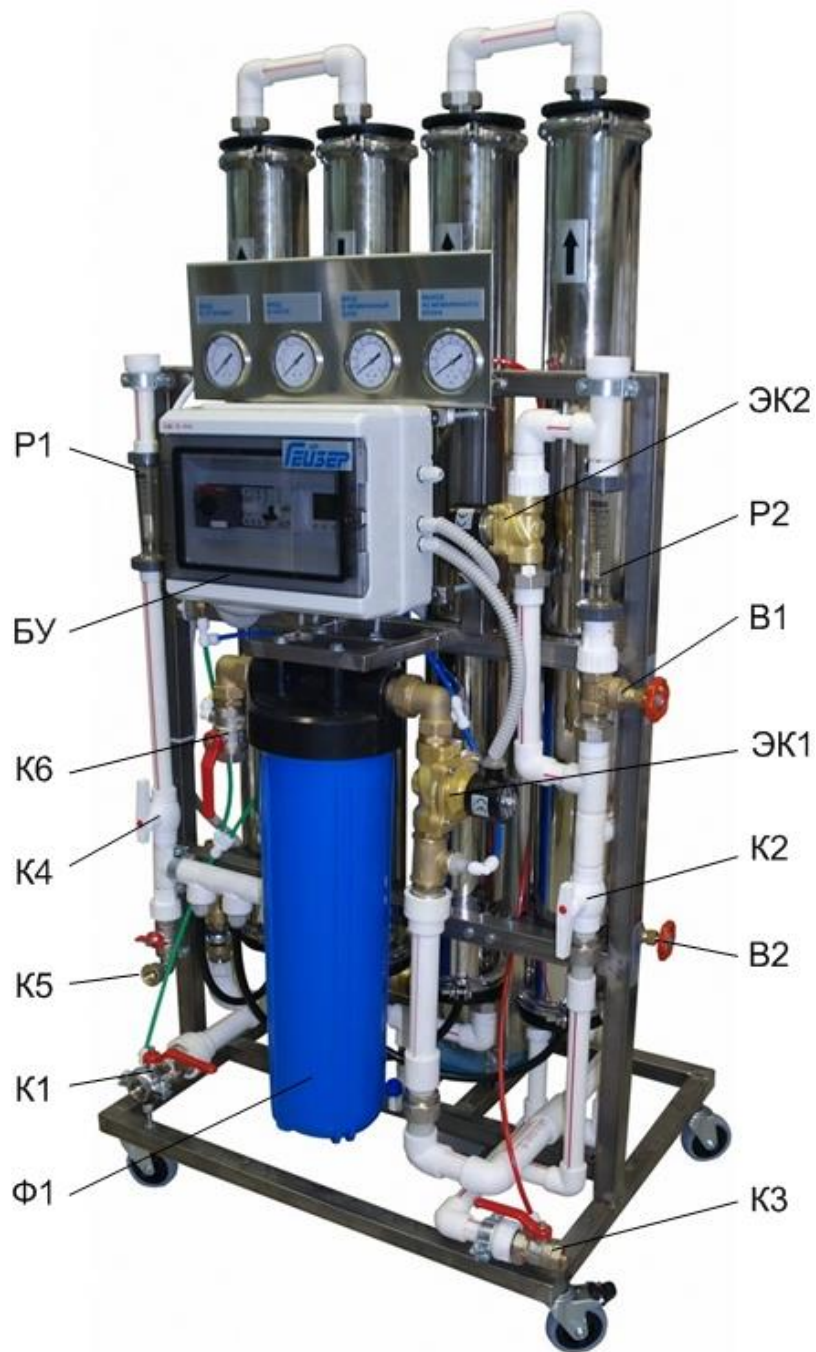
Рис.1 Общий вид установки (с лицевой стороны).
