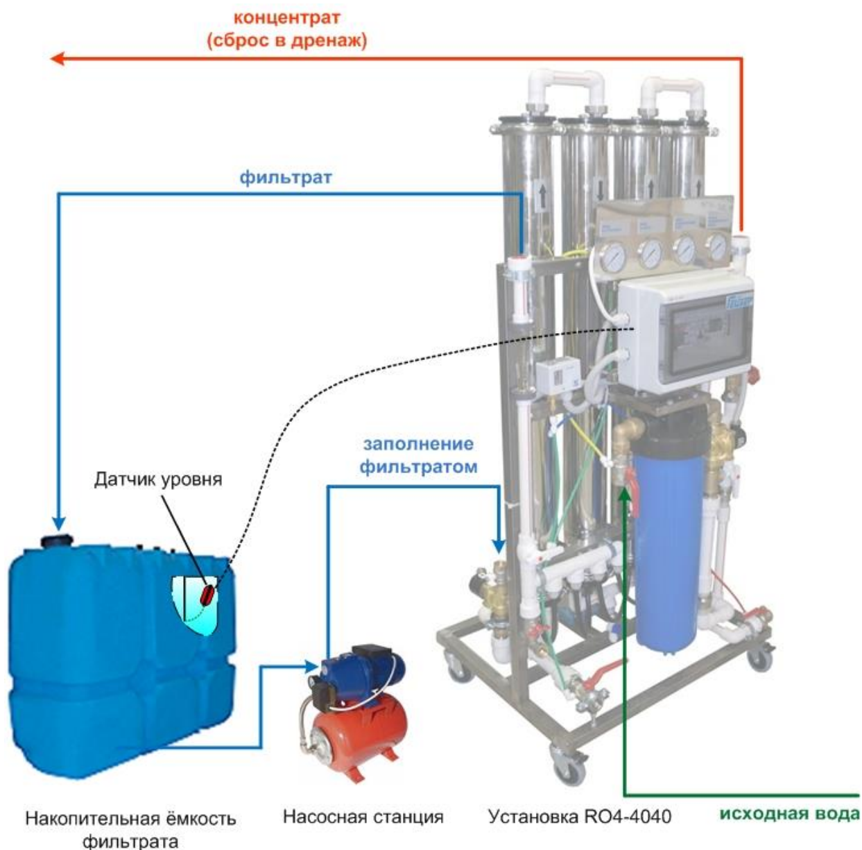
Рис. 6 Подключение трубопроводов к установке.
