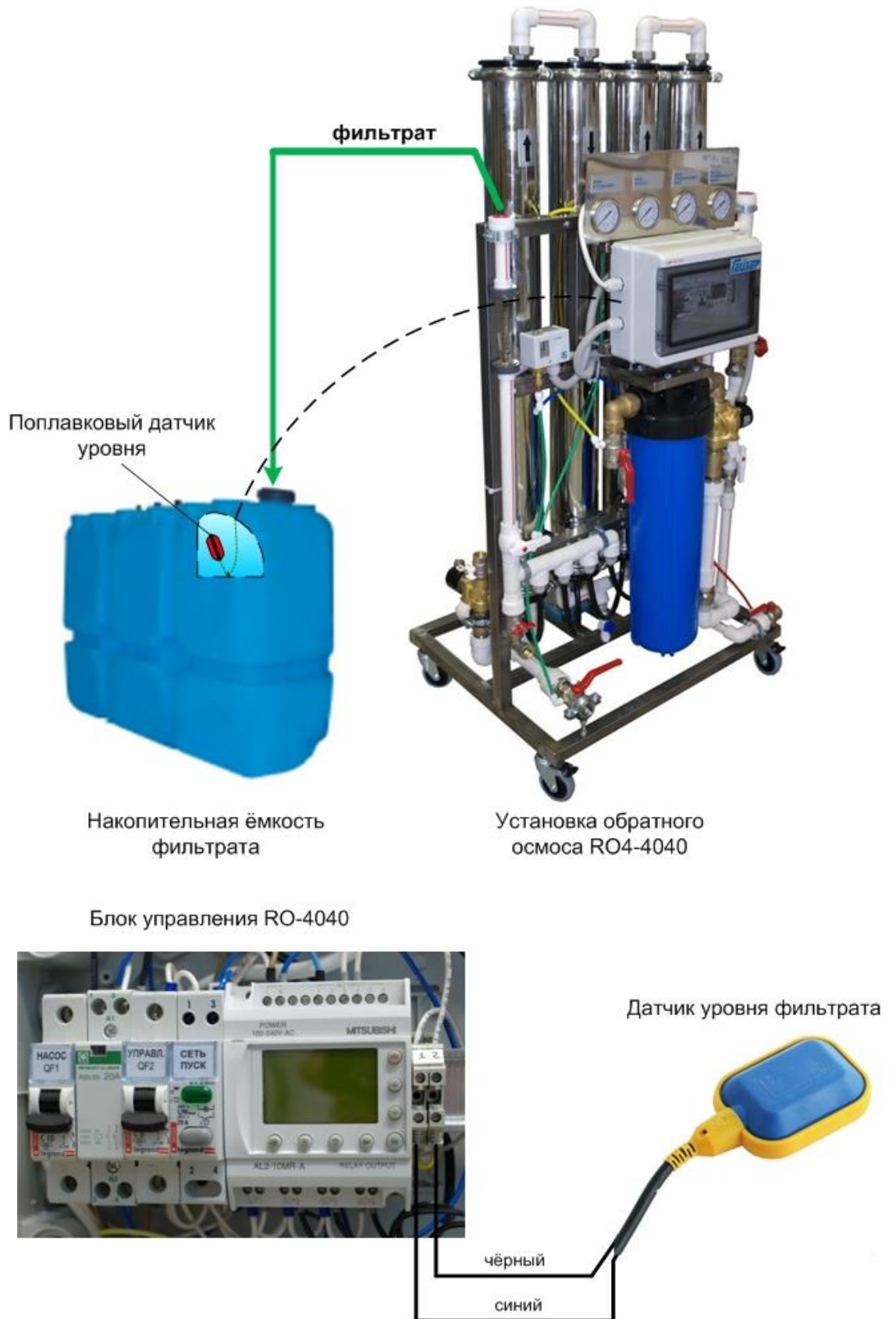
Рис.5 Подключение одного датчика уровня к установке.
