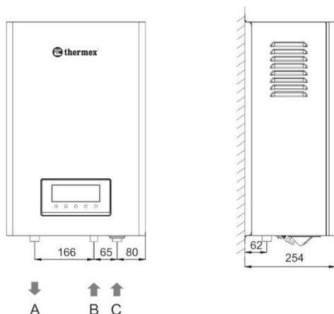
Рис. 7. Присоединительные размеры
