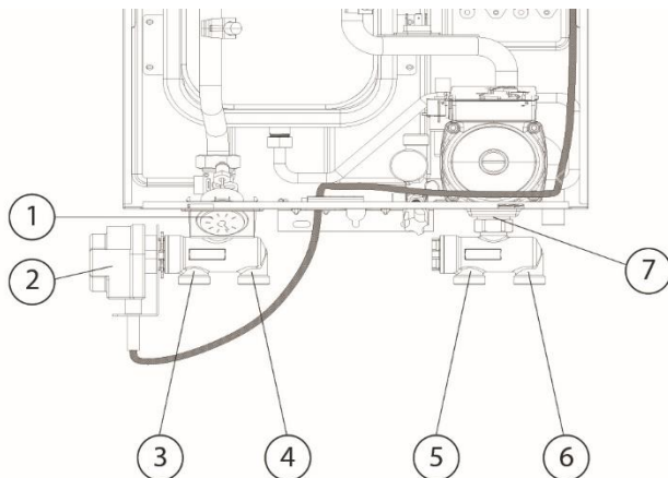
Рис.15. Присоединение трехходового клапана
