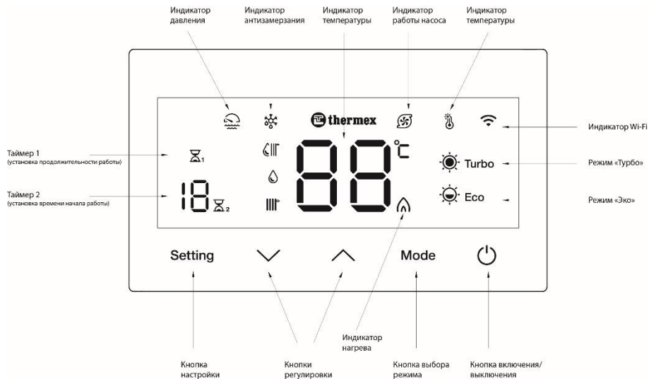
Рис. 3. Панель управления
