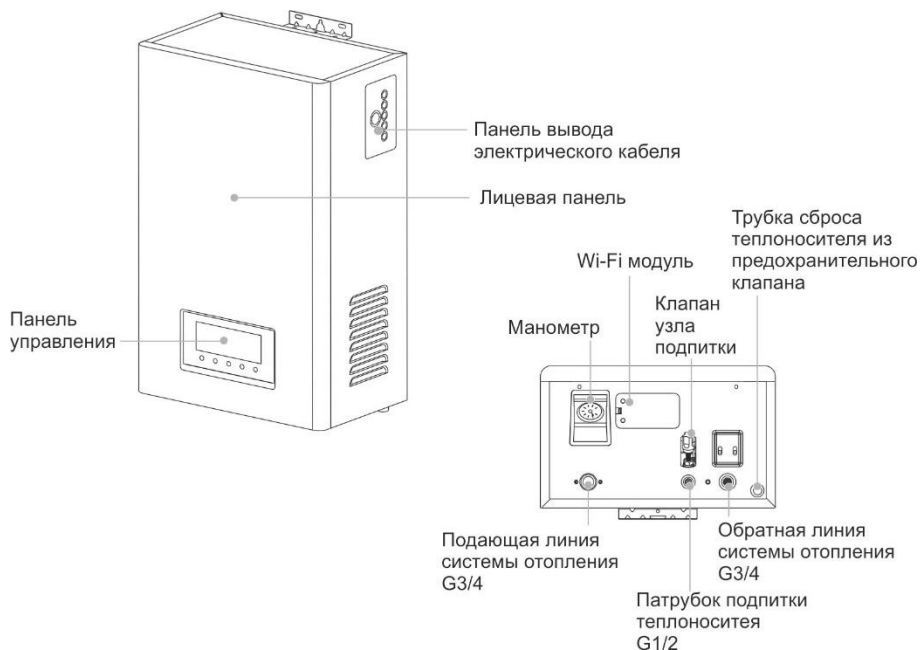
Рис. 1. Конструкция изделия
