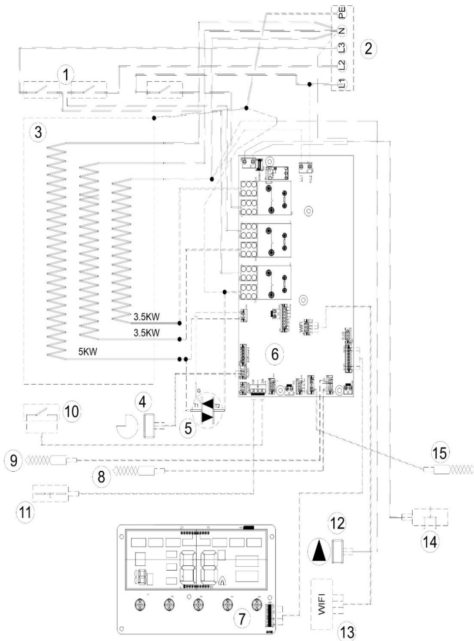
Рис. 19. Электрическая схема THERMEX Skif 5-12 Wi-Fi
