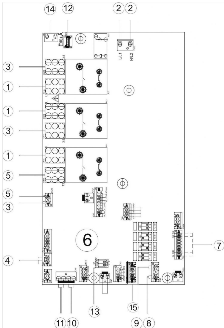
Рис. 20. Электрическая схема основной платы управления
