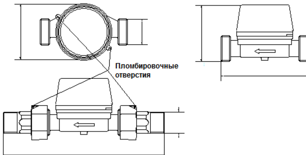
Рисунок 1. Счетчики воды
