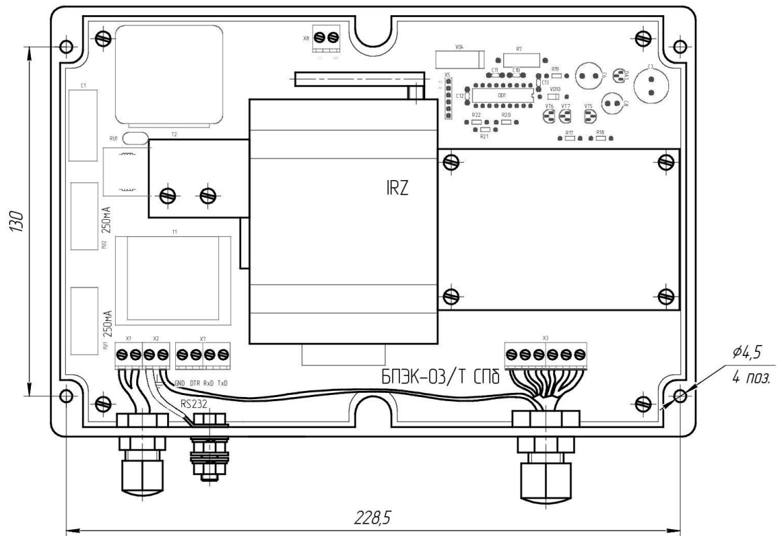
Рисунок 3.1 - Крепежные размеры блока питания БПЭК-03/Т СПб
