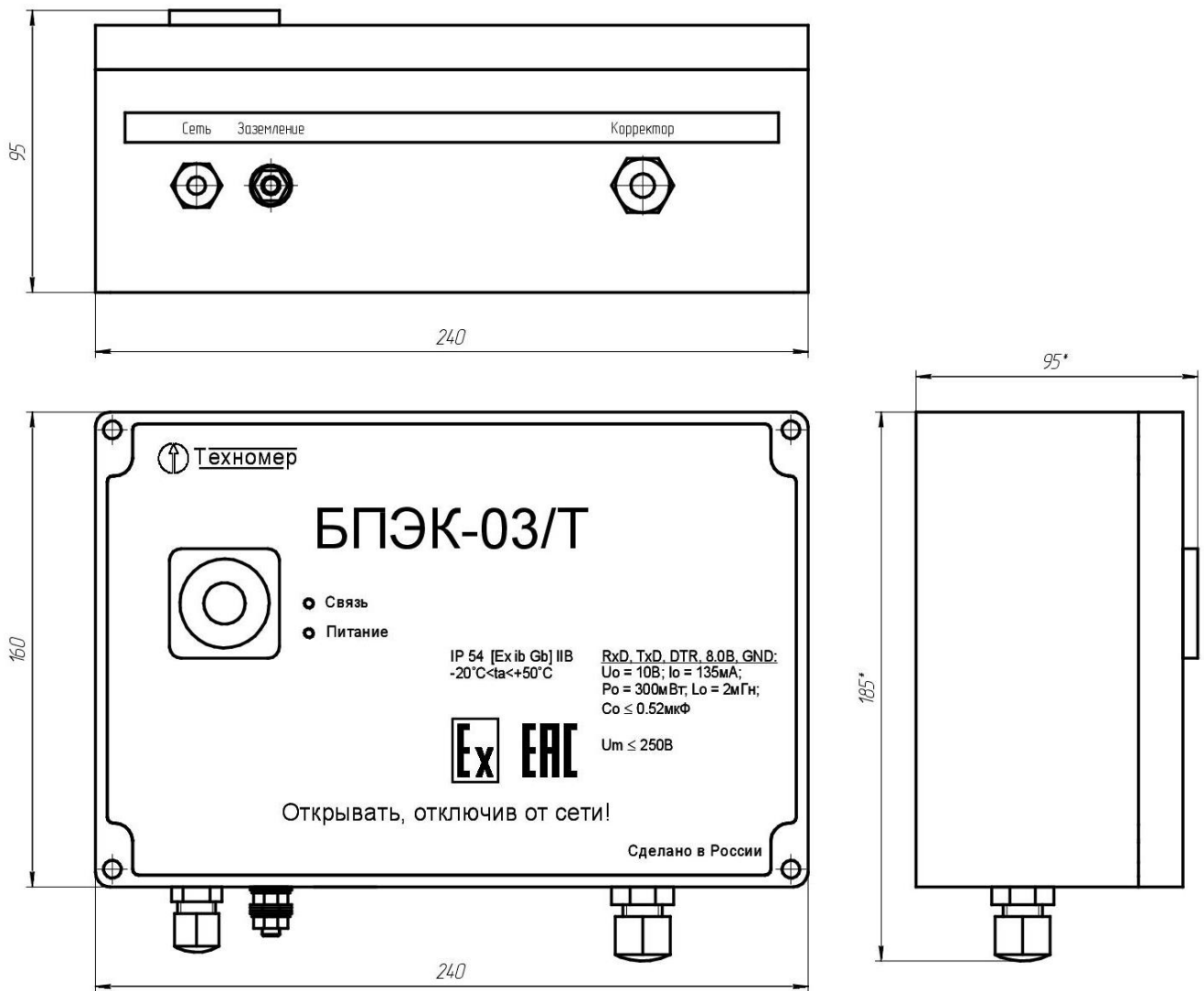
Рисунок 1.1 - Габаритные размеры блока питания БПЭК-03/Т СПБ
